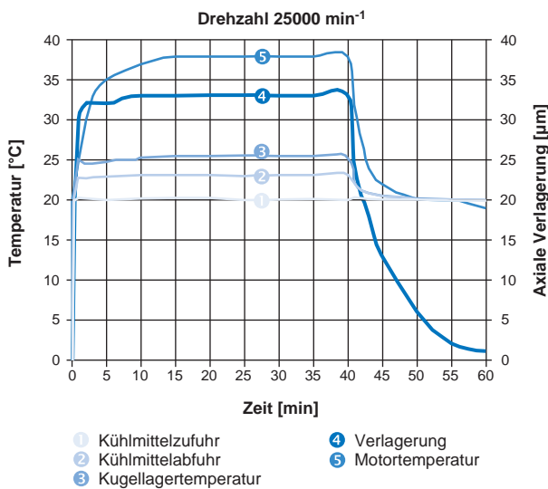
Diagramm zur Veranschaulichung der axialen Wellenverlagerung bei einer Spindeldrehzahl von 25000 min -1 .
