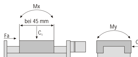
Zulässige Belastungen domiLINE 30 Maximum loads domiLINE 30
