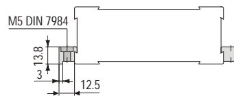
Befestigungssatz B Fastening set B
