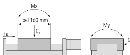
Zulässige Belastungen domiLINE 120 Maximum loads domiLINE 120
