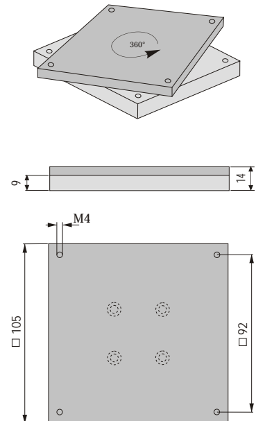
Dreheinheit Rotational unit
