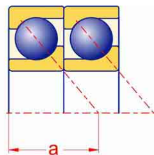
Tandemanordnung Tandem arrangement
