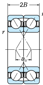
Front-to-Front DF
