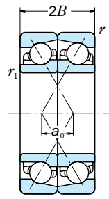
Front-to-Front DF
