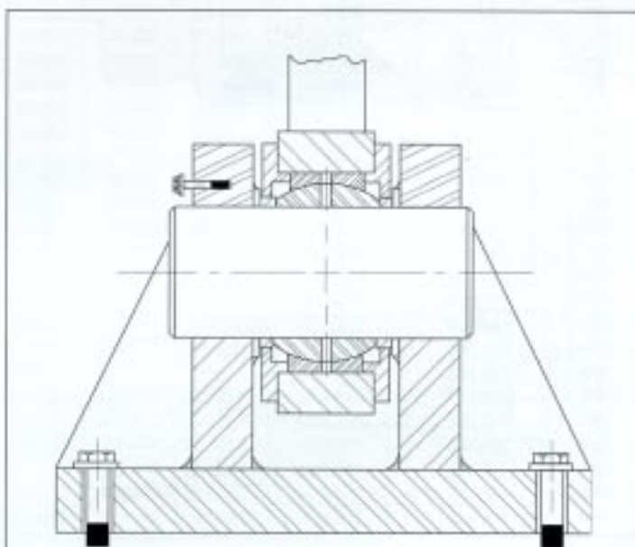
Hinge Pin
