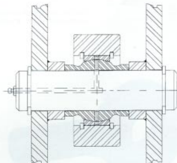
Tie Rod
